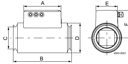
Габаритный чертеж датчика расхода Альфа Laval TE67A6XXXXXXXX
